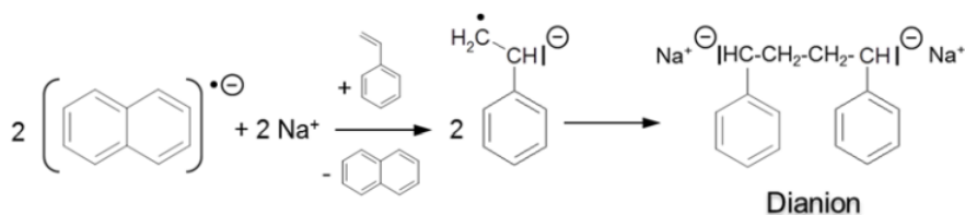
Abb. 3: Die Abbildung zeigt den Initiierungsschritt von Styrol mittels eines Alkalimetallnaphthaliden.[1]
